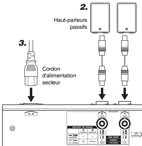
Panneau arrière (Reportez-vous à la page 14.)
