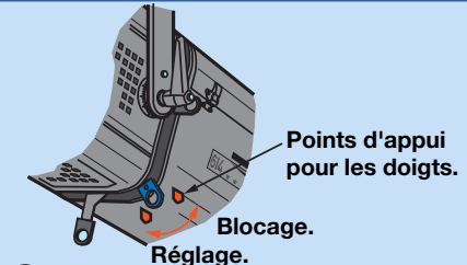
4 Blocage des couteaux.
