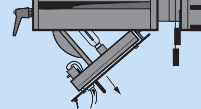
8 Accès lampe (600SX)
