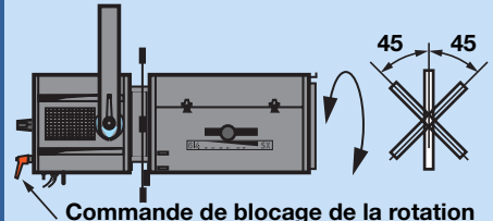
3 Ensemble fenêtre et zoom tournant. 3 Commande de blocage de la rotation du zoom.
